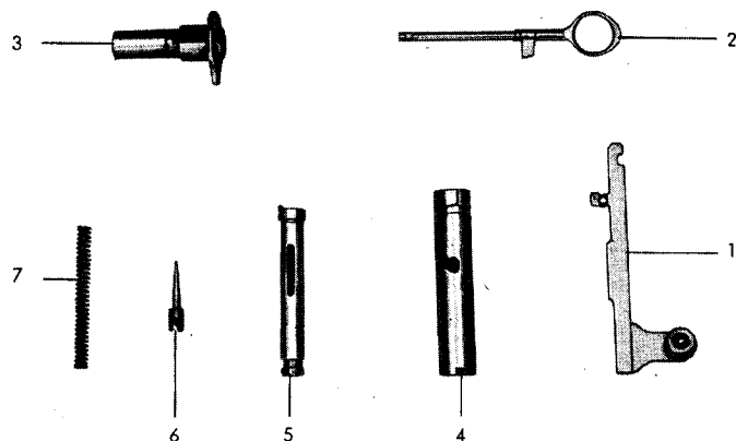
Bild 3 Verschluß zerlegt
