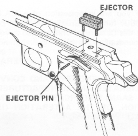
Illust. No. 13— EJECTOR & EJECTOR PIN
